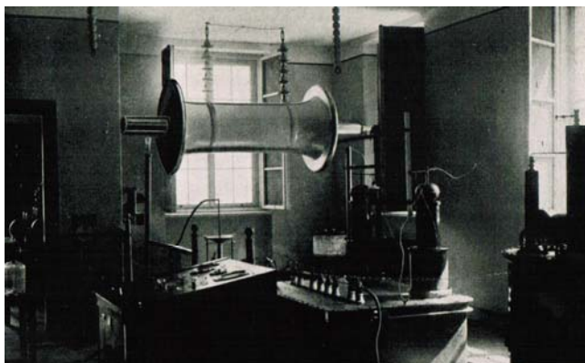
Rys. 2. Fotografia laboratorium wysokich napięć wykonana przed rokiem 1930; w centralnym punkcie jest zawieszony kondensator powietrzny o pojemności 50 pF a po prawej stronie widoczny fragment transformatora o napięciu 150 kV [13]
